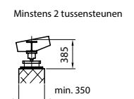
Detail Y
