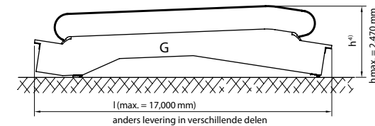
Transportafmetingen
